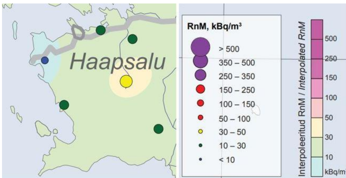
Joonis 20. Radooni sisaldus pinnaseõhus Haapsalu linna territooriumil. Allikas: Eesti pinnase radooniriski ja looduskiirguse atlas, seisuga 21.06.2019
